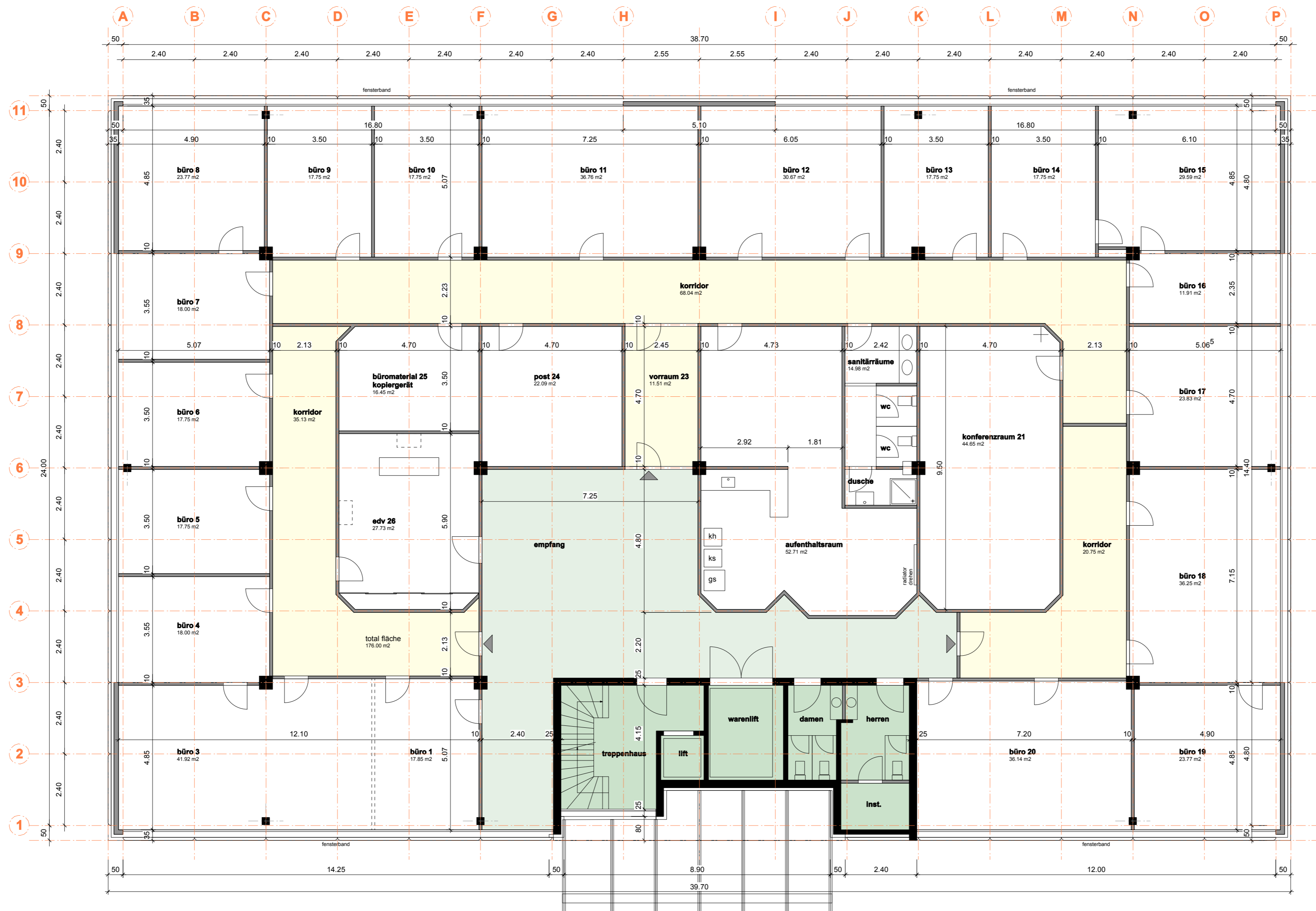
GRUNDRISS 1. OBERGESCHOSS
