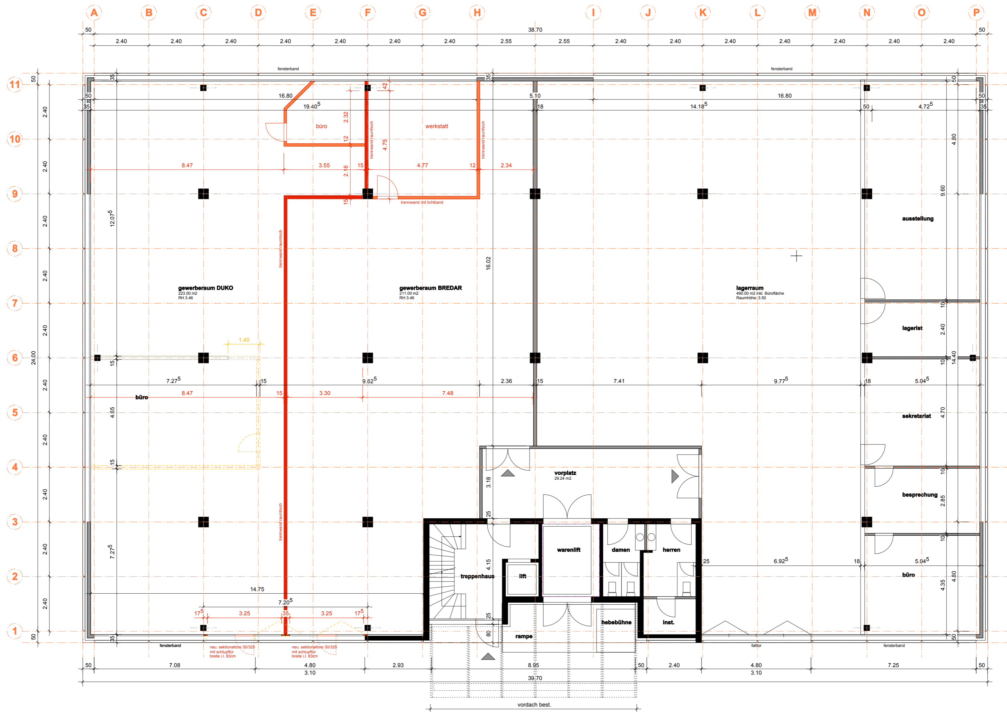
GRUNDRISS ERDGESCHOSS
